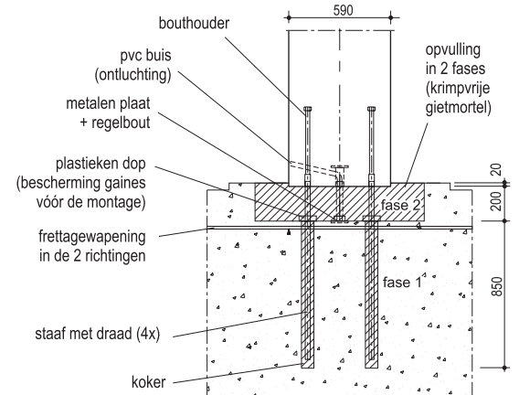
AANSLUITING KOLOM-FUNDERING
