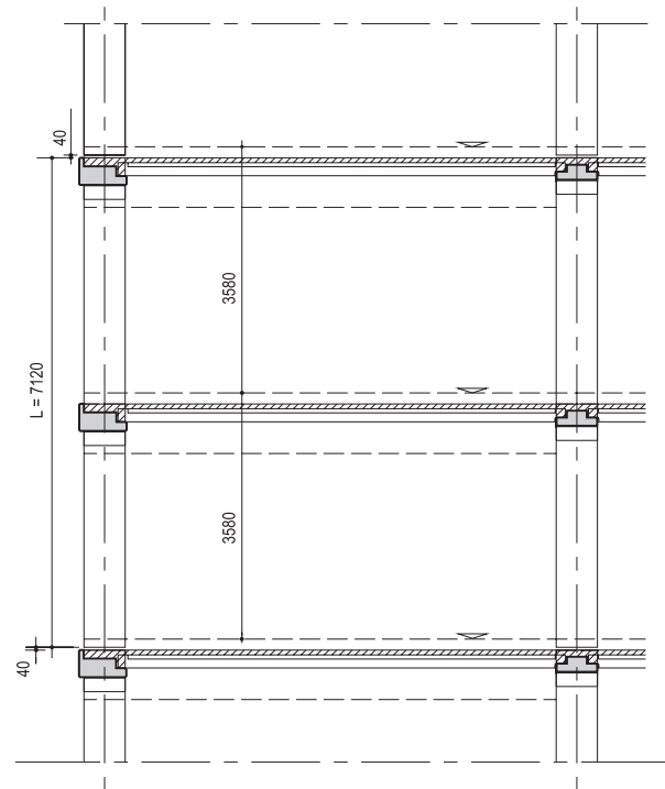
SNEDE A-A
