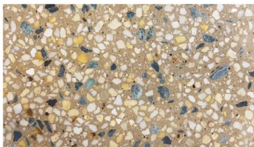
Foto referentiestaal gepolijste cementbetonverharding.
