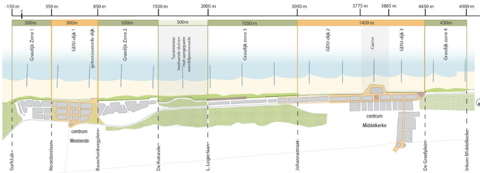
Toekomstige GDU-dijk: stedelijke zone (40% van zeedijk). 1,5 km dijk in centrum Middelkerke en 500m dijk in centrum Westende
