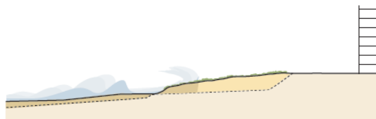
Toekomstige grasdijk: residentiële zone (60% van zeedijk)
